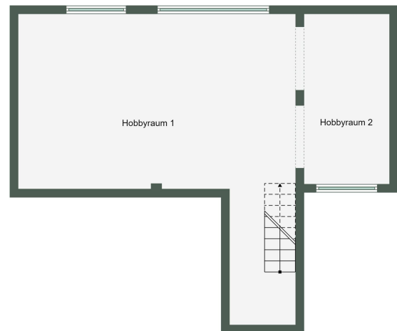
Grundriss Souterrain
